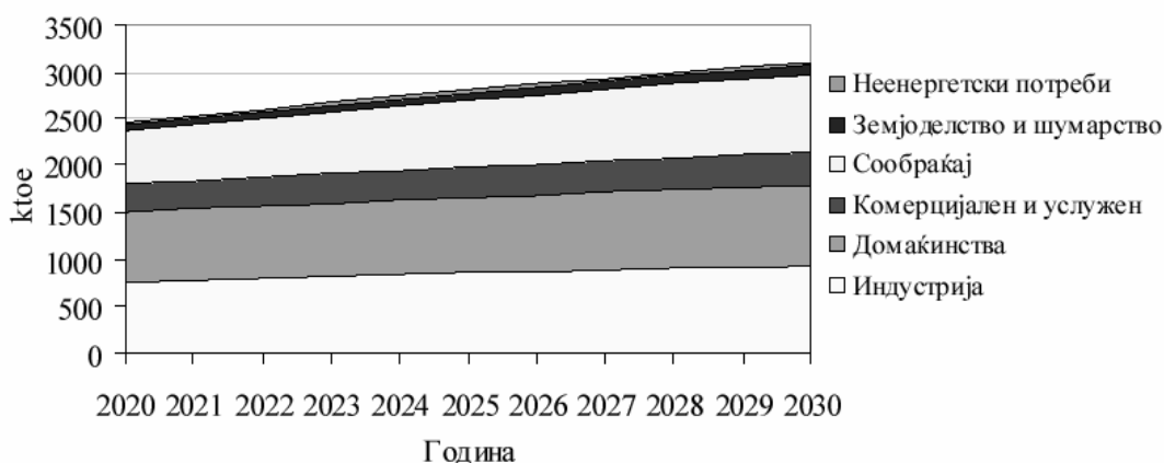
Слика 10.1.1.2. Потребите од вкупна финална енергија до 2030 година според сценариото со засилени мерки за енергетска ефикасност (ktоe)
