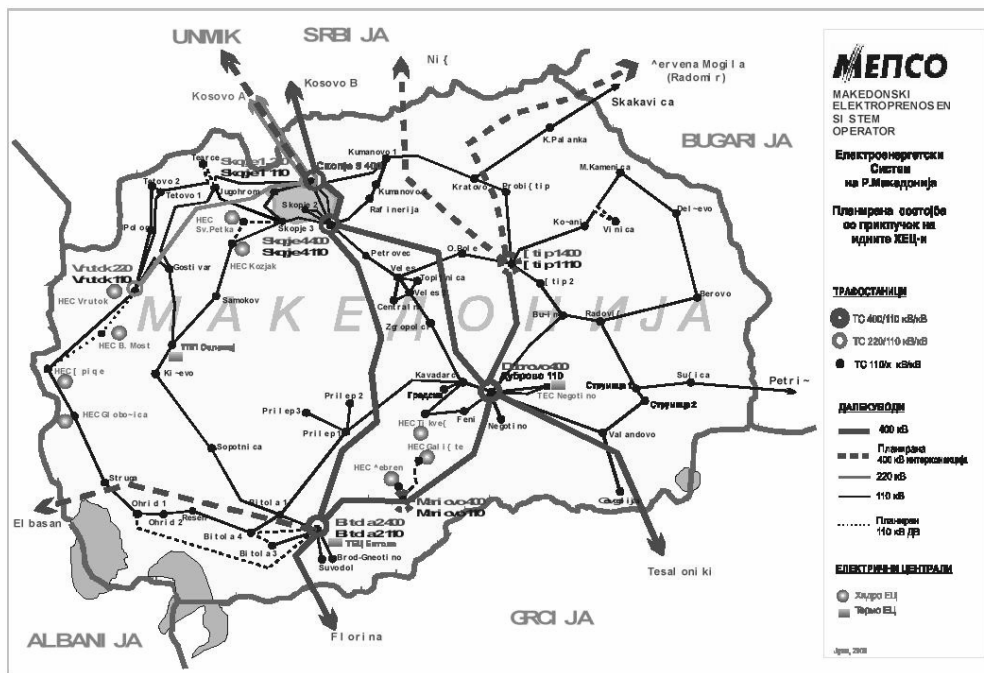
Слика 3.2.2.1. Постојни и планирани објекти на преносниот систем на РМ
