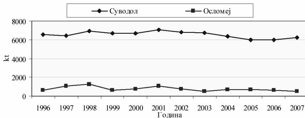
Слика 4.2.1.1. Потрошувачка на лигнит од домашно производство 44
