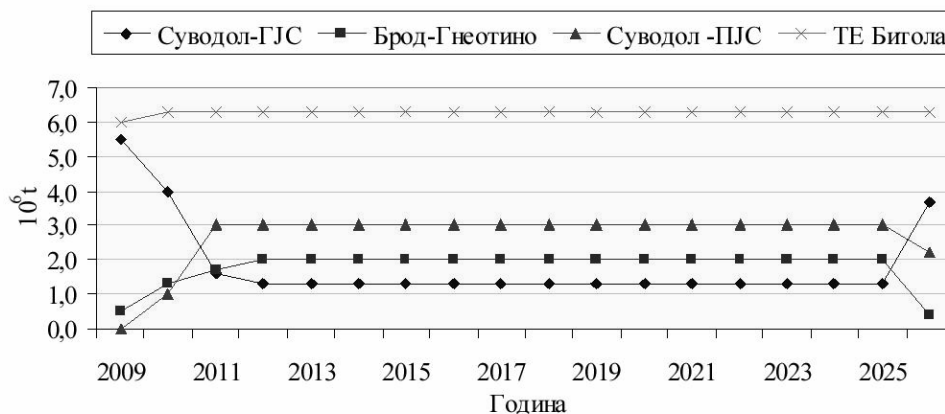
Слика 6.3.1.1. Динамика и количини на произведен јаглен од поедини копови за потребите на ТЕ Битола 1, 2 и 3, во периодот од 2009-2026 година
